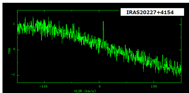
図 1 2014 年 12 月の単一鏡観測で得られた \text{H}_2\text{O} メーザーのスペクトルの一例。(左) 長周期変光星 Z Cyg のスペクトル。(右) 超新星残骸 SNR G078.2+02.1 付近にある IRAS 20227+4154 のスペクトル。
