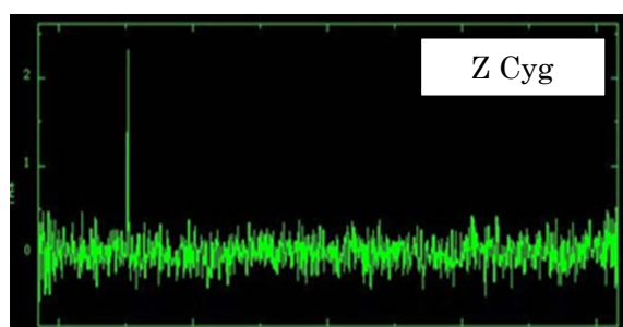
図 1 2014 年 12 月の単一鏡観測で得られた \text{H}_2\text{O} メーザーのスペクトルの一例。(左) 長周期変光星 Z Cyg のスペクトル。(右) 超新星残骸 SNR G078.2+02.1 付近にある IRAS 20227+4154 のスペクトル。
